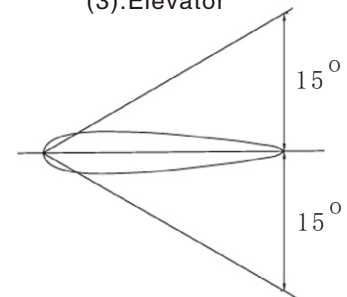
(3). Elevator
