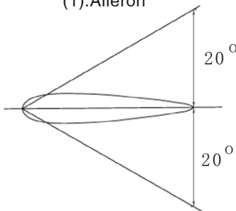
(1). Aileron
