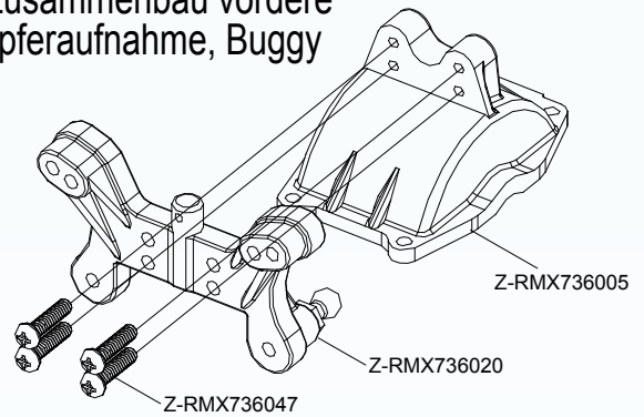
12. Shock Plate Assembly 12. Montage Dämpferaufnahmen
