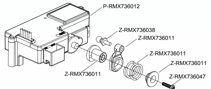
16. Servo Saver Assembly 16. Zusammenbau Servo Saver
